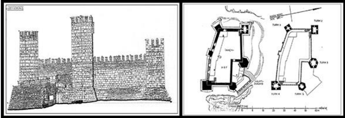
Görsel 4: Çandarlı Kalesi'nin Plan ve Görünüşü
